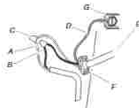
A. Conducteurs blancs B. Conducteurs noirs C. Connecteur de fils homologues UL D. Fil de terre vert (ou nu) E. Câble d'alimentation du domicile ou cordon d'alimentation F. Serr-câbles "Y" homologues UL ou CSA G. Vis de terre à la terre
