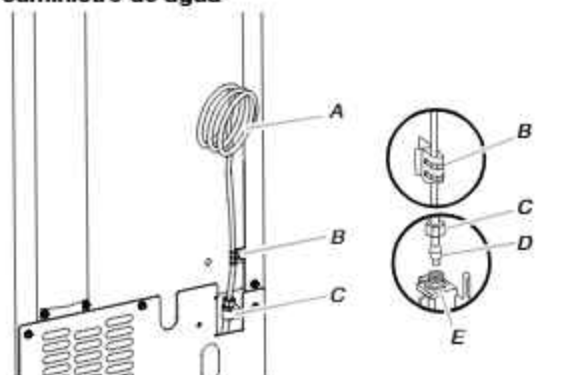
A. Tubería de cobre de 1/4"
