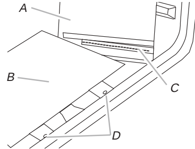
A. Miroir B. Répartiteur de flammes C. Réflexissement de la flamme D. 2 vis
