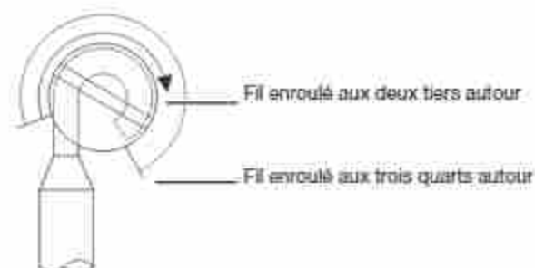
Dénuder l'isolation et enrouler le fil Illustration : 1
