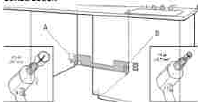
A. Emplacement optionnel B. Emplacement standard
