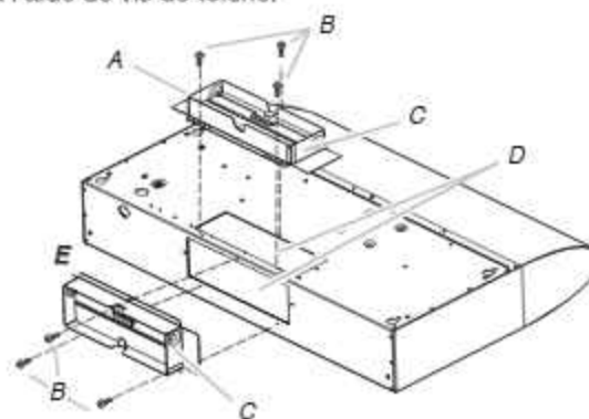
A. Conduit vertical B. Vis de tôle C. Axe de charnière D. Opercules arrachables du conduit d'évacuation E. Conduit horizontal
