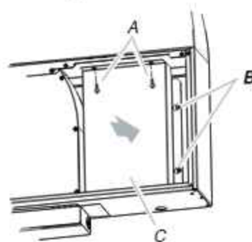
A. Vis B. Pattes de montage C. Couvercle du boîtier de connexion
