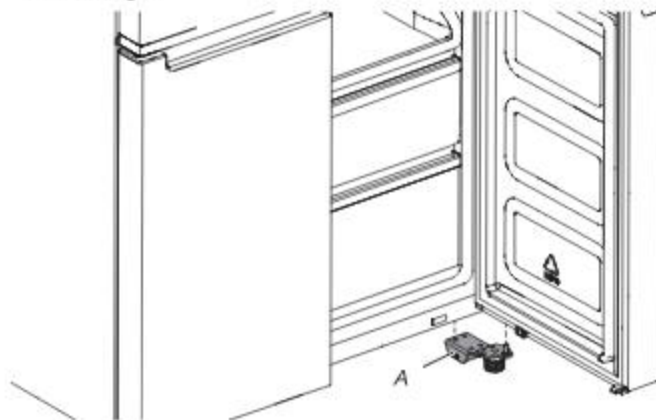
A. Bisagra inferior
