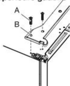
Couvercle de charnière supérieure gauche
