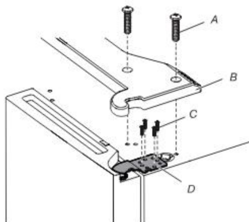
A. Vis du couvre-charnière supérieur B. Couvre-charnière supérieur C. Vis à tête creuse de 5 mm D. Charnière supérieure
