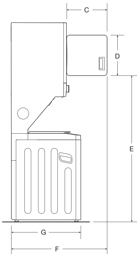
VUE LATÉRALE
