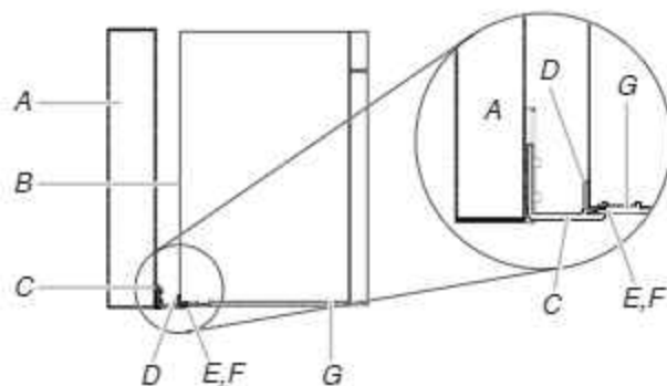
A. Mur B. Arrière du four à micro-ondes C. Ensemble de montage de bourrelet D. Butée d'accrochage E. Crochet F. Trou noir de la plaque inférieure G. Plaque inférieure
