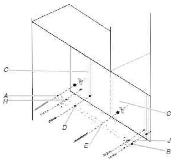
A et B. Deux trous d'extrémité C. Montants muraux D, E, H, et J. Quatre trous pour tirefonds
