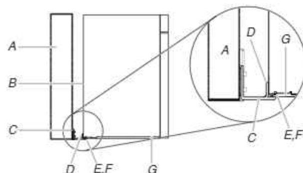
A. Pared B. Parte trasera del horno microondas C. Kit de montaje sobresaliente D. Tope colgante E. Gancho colgante F. Orificio trasero de la placa inferior G. Placa inferior
