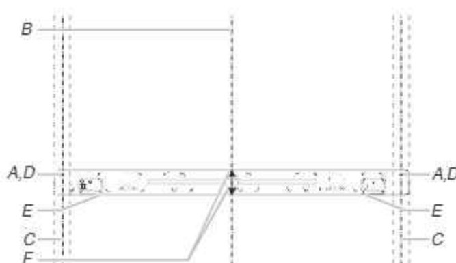
Montant de cloison à la position des trous d'extrémité Illustration 4
