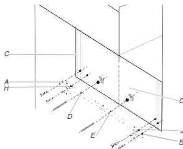
A et B. Deux trous d'extrémité C. Montants muraux D, E, H, et J. Quatre trous pour tirefonds
