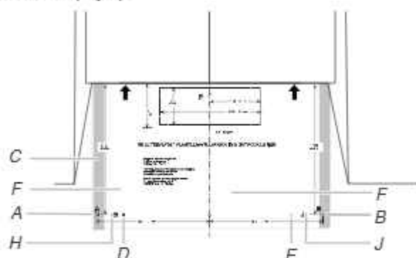
A y B. Dos orificios de extremo C. Viga de pared D, E, H y J. Cuatro orificios para tirafondos F. Plantilla de pared
