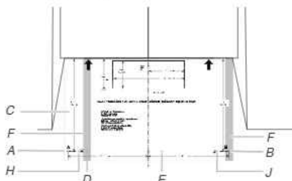
A. Orificios de extremo B, E, H y J. Cinco orificios para tirafondos C. Plantilla de pared F. Viga de pared
