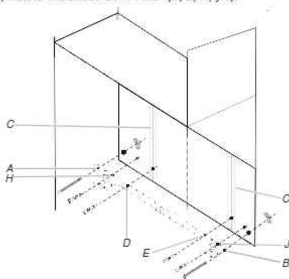
A y B. Dos orificios de extremo C. Vigas de pared D, E, H y J. Cuatro orificios para tirafondos
