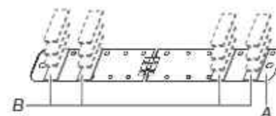
A. Plaque de montage B. Entretoise de 1/16 po (1,58 mm) d'épaisseur
