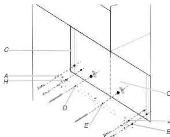
A y B. Dos orificios de extremo C. Vigas de pared D, E, H y J. Cuatro orificios para tirafondos
