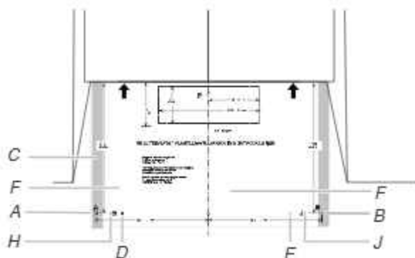
A y B. Dos orificios de extremo C. Viga de pared D, E, H y J. Cuatro orificios para tirafondos F. Plantilla de pared
