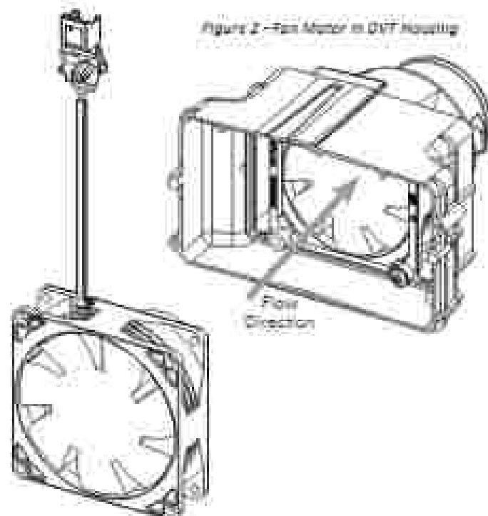
Figure 2 - Fan Motor
