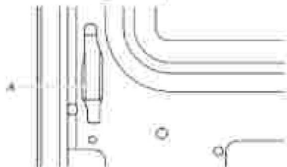
A. Ranura en la cavidad del horno para la muesca de bisagra de la puerta
