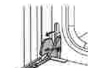
Traba de bisagra de la puerta del horno en posición destrabada
