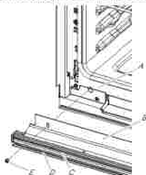
A. Châssis du four B. Déflecteur C. Évent du four D. Ongle de l'évent E. Vis no 5-16 x 3/8 po (9,5 mm)
