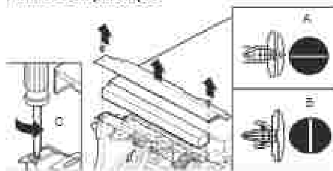
A. Déverrouillé C. 1/4 de tour E. Verrouillé
