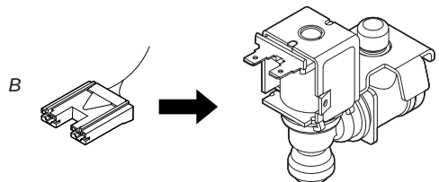
Adaptación del conector del mazo de cables a la válvula
