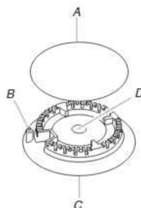
Brûleur standard et brûleur à double flamme
