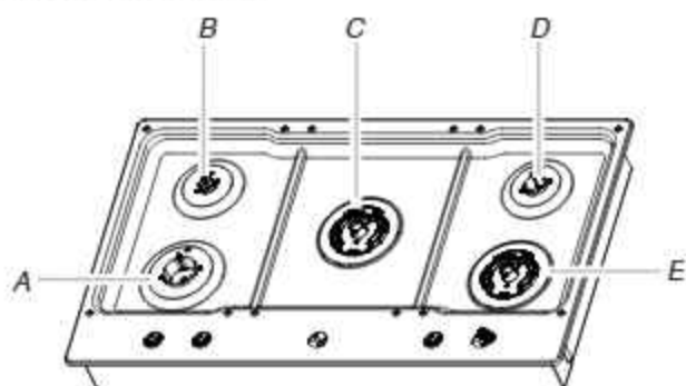
A. Avant gauche B. Arrière gauche C. Centre D. Arrière droit E. Avant droit
