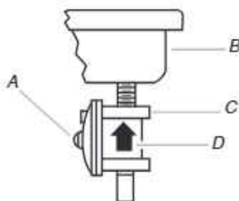
A. Chapeau de l'ouverture d'accès B. Arrière de la table de cuisson C. Détendeur D. Sens de circulation du gaz
