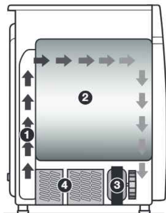
Unité de pompe à chaleur HybridCare™
