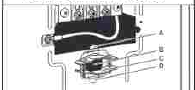
Conector de 4 hilos (tipo NEMA 14-30R)
