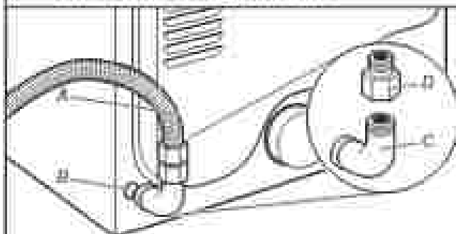
A. Raccord flexible de gaz de 28 po B. Conduit de la longueur de 30 po C. Guide de 1/4 po par 3/8 po D. Adaptateur entre le conduit et le joint conique de 3/8 po
