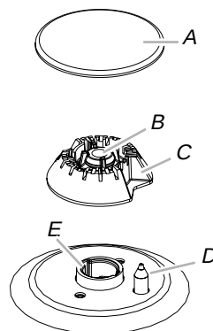
A. Chapeau de brûleur D. Electrode d'allumage B. Tube d'arrivée de gaz E. Support d'injecteur à orifice C. Base du brûleur
