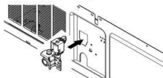
Insertado de la válvula
