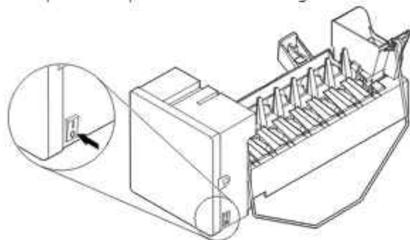
Apagado de la fábrica de hielo (interruptor basculante)
