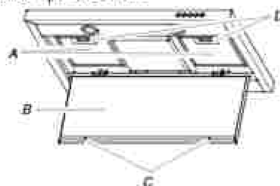
A. Filtres métalliques B. Panneau en acier inoxydable C. Filtres de retenue (2) D. Loquets à ressort (2)
