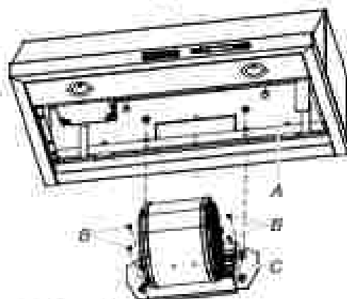
A. Intérieur de la hotte (verso) B. 4 vis de 4,2 x 8 mm C. Ensemble du support de montage du moteur du ventilateur arrière
